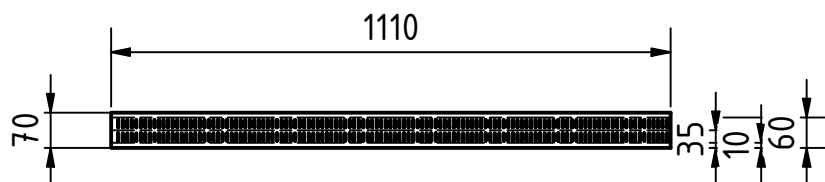
NDV-3102 Крышка луча 1, s=0.8 1 шт. на NDV-3100; 4 шт. на проект
