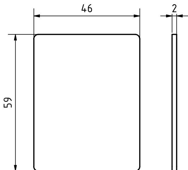
NDV-3002 Заглушка луча, s=2.0 1 шт. на NDV-3100; 24 шт. на проект
