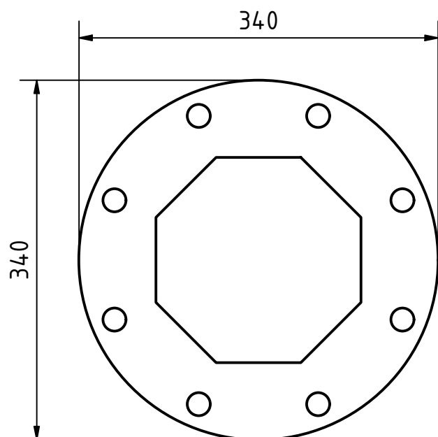
NDV-1103 Фланец центра нижний, s=5.0 1 шт. на NDV-1000; 1 шт. на проект
