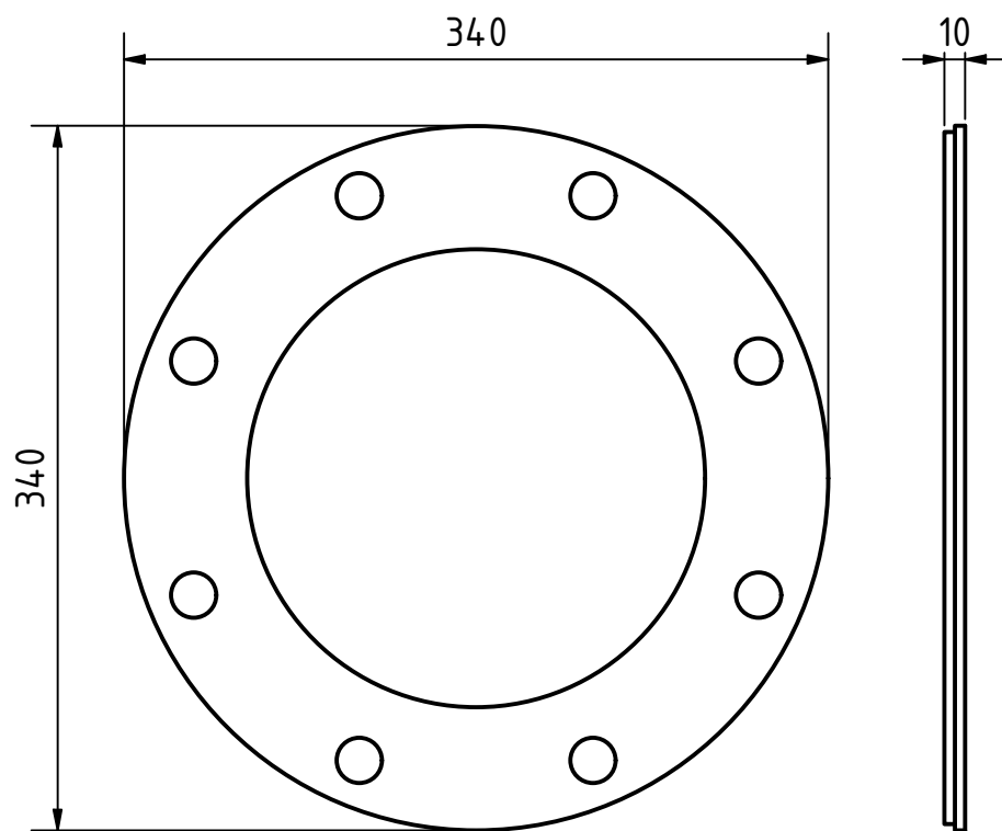
NDV-4000 Фланец трубы DN200 1 шт. на проект
