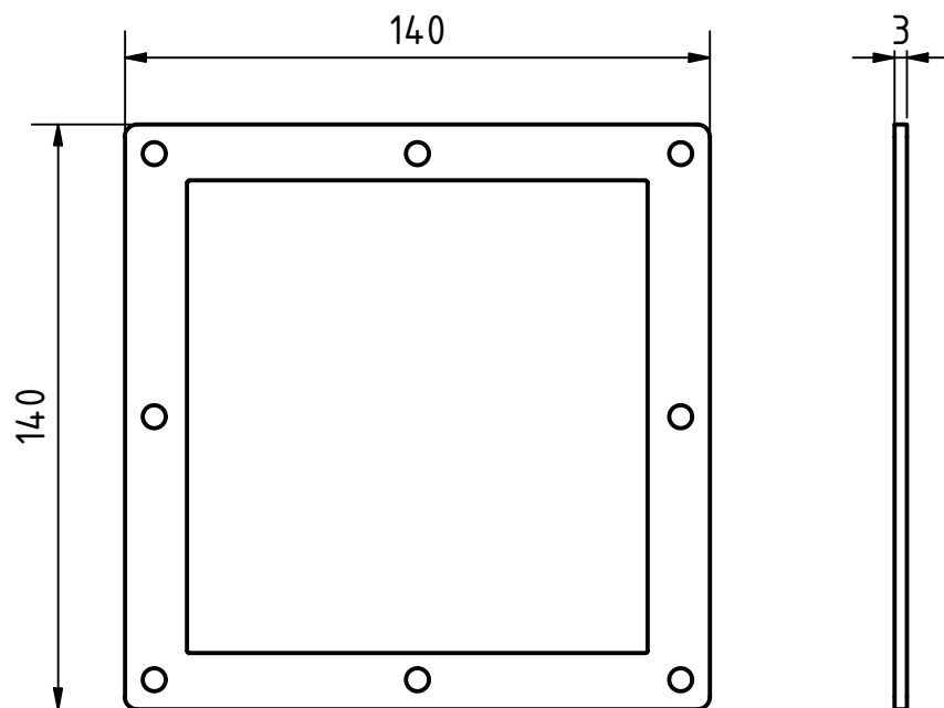
NDV-2103 Фланец коллектора, s=3.0 1 шт. на NDV-2000; 4 шт. на проект
