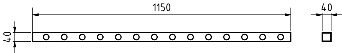
NDV-3101 Труда луча 1
