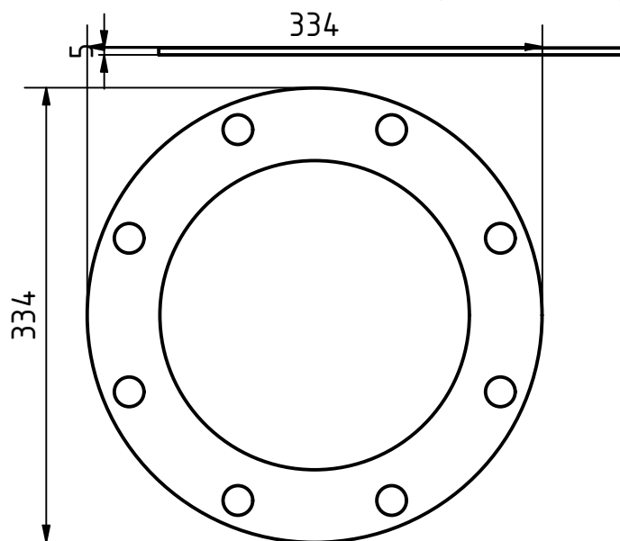
NDV-4101 Фланец трубы нижний, s=5.0
